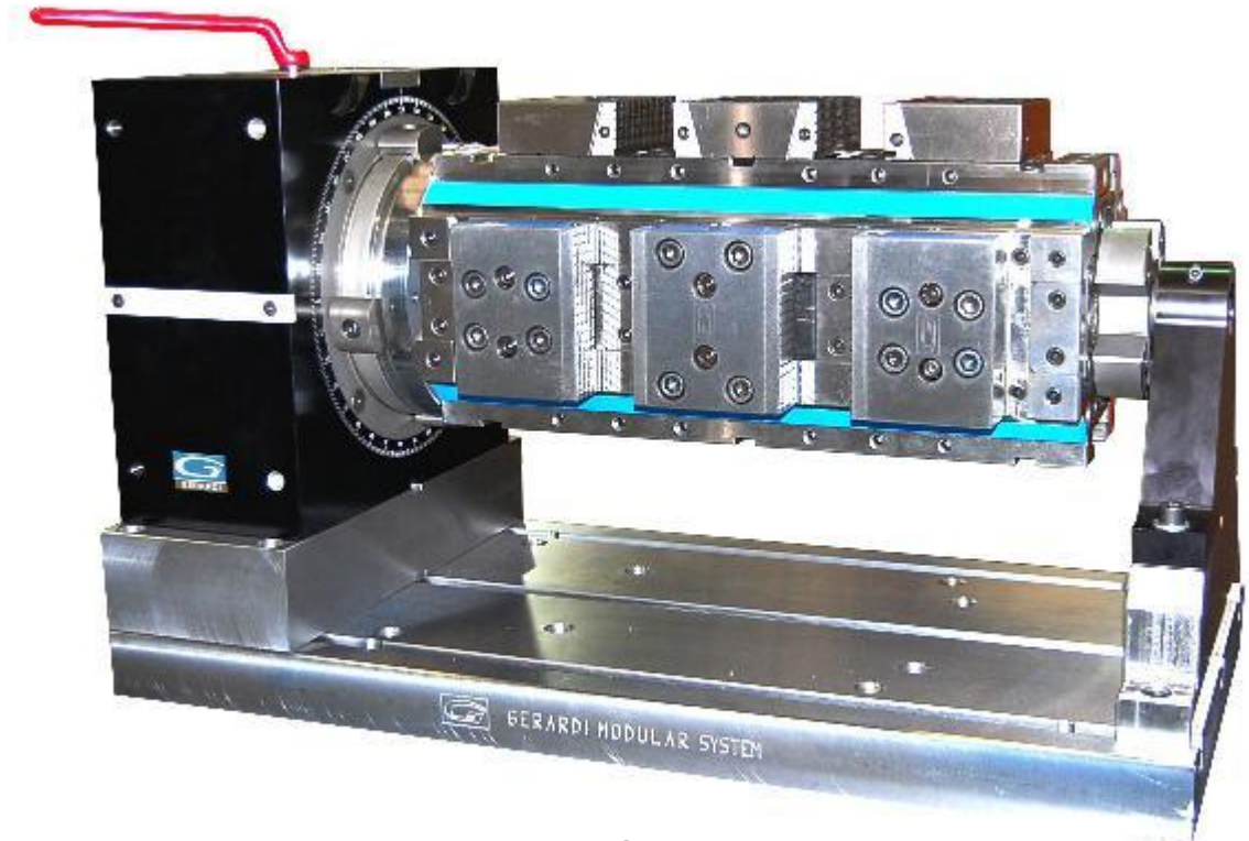
Ejemplo de Divisor con cubo FMS y contrapunto
